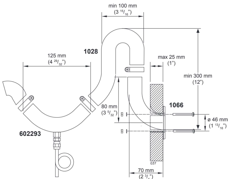
Zijkant doorlaat 1066
